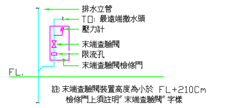
末端查驗管裝置示意圖
